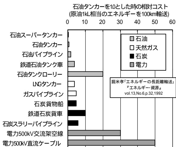
図1 エネルギー輸送のためのコスト
